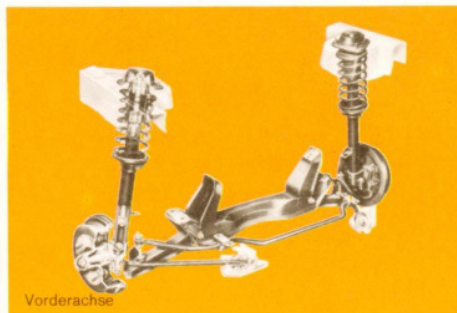
Vorderachse
