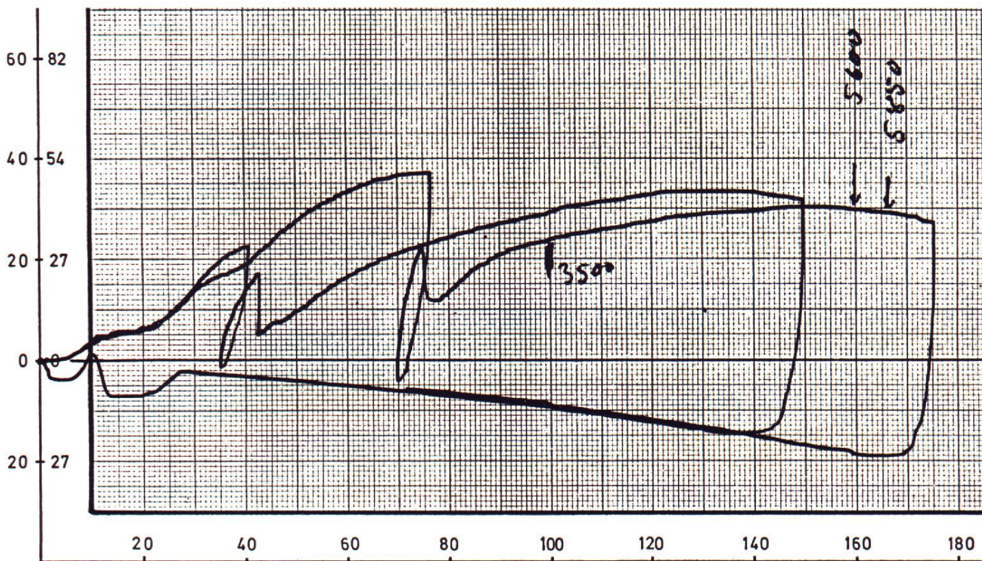
Leistungsdiagramm „Micra“
